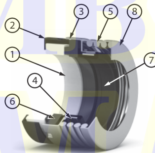
Figura 1: Sello seccionado
